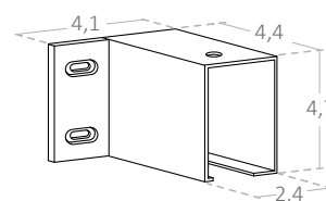
Esquadra de parede Wall support
