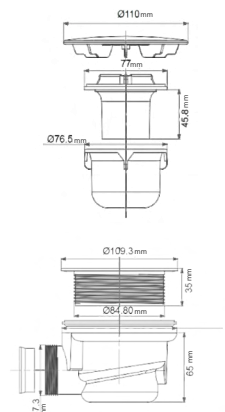
Válvula Vlave
