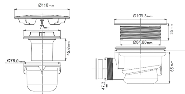
Válvula Valve
