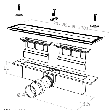
Válvula Valve
