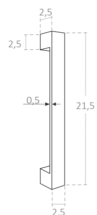
Puxador Handle
