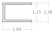
Perfil de parede do vidro móvel Mobile glass wall profile
